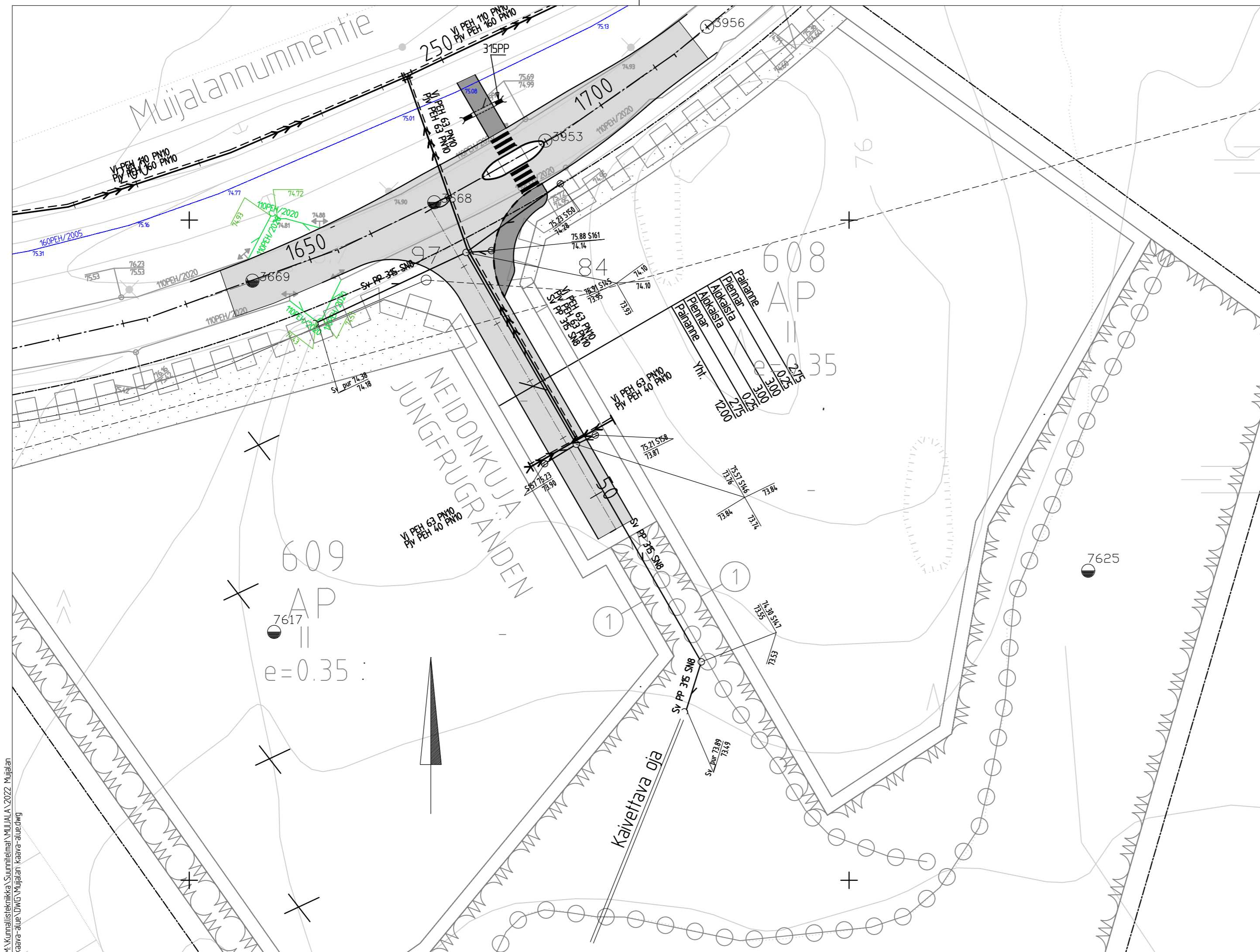
Sadevesiviemärien yhdysputket 160 PP-SN8
