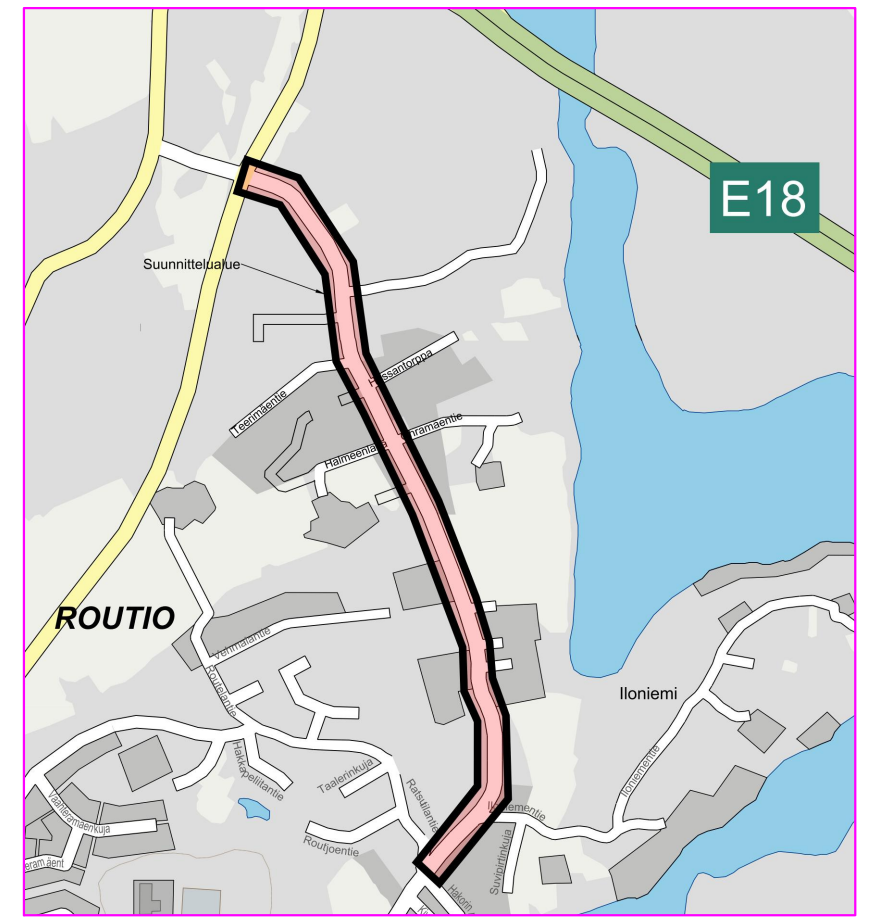
Sadevesiviemärien yhdysputket 160 PP-SNB Koordinaatti- ja korkeusjärjestelmä ETRS-GK24/N60
