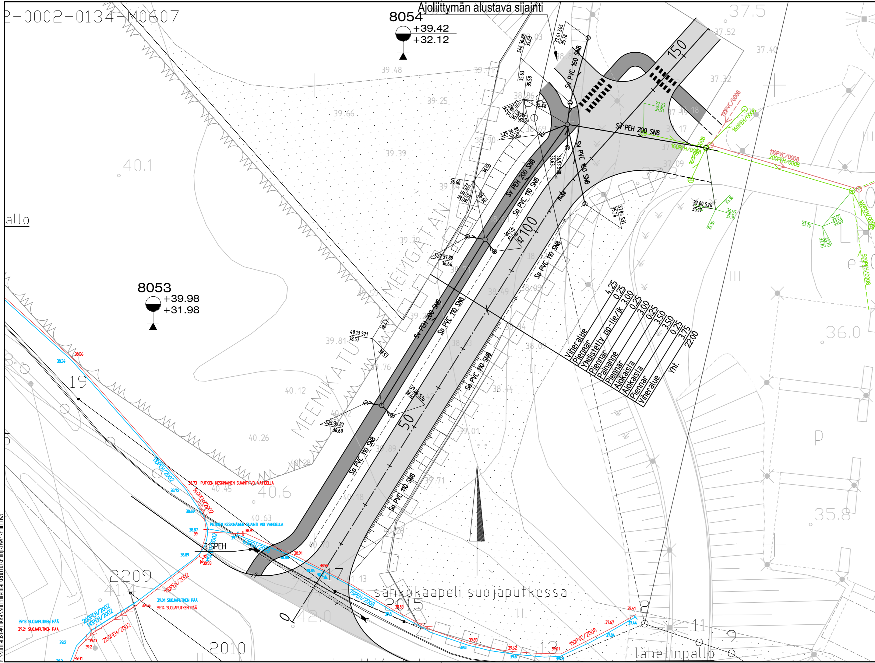
Sadevesiviemärien yhdysputket 160 PP-SN8 Koordinaatti- ja korkeusjärjestelmä ETRS-GK24/N2000
